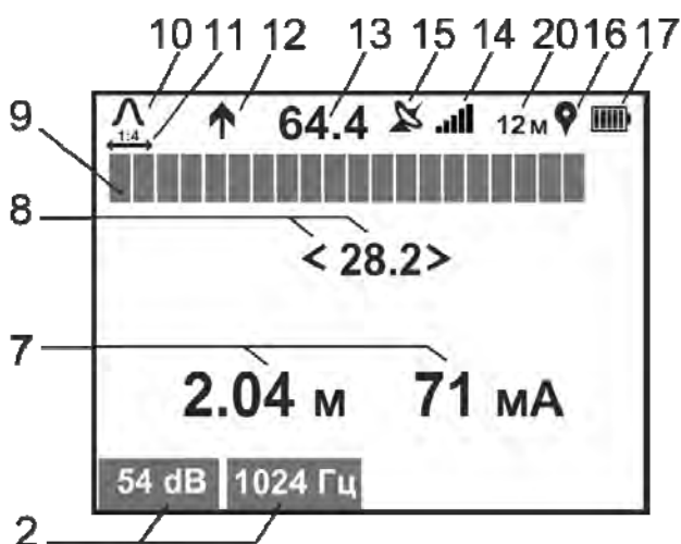
Рисунок 3.2 – Индикация приемника в режиме «ТРАССА»
