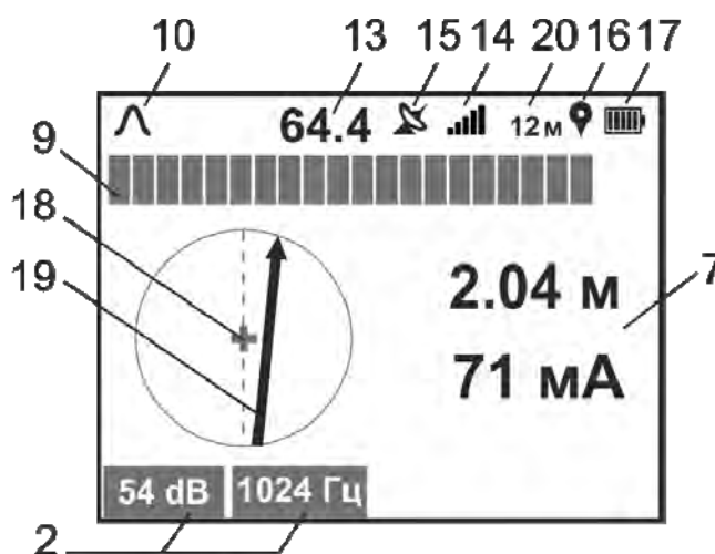
Рисунок 3.2 – Индикация приемника в режиме «ТРАССА»
