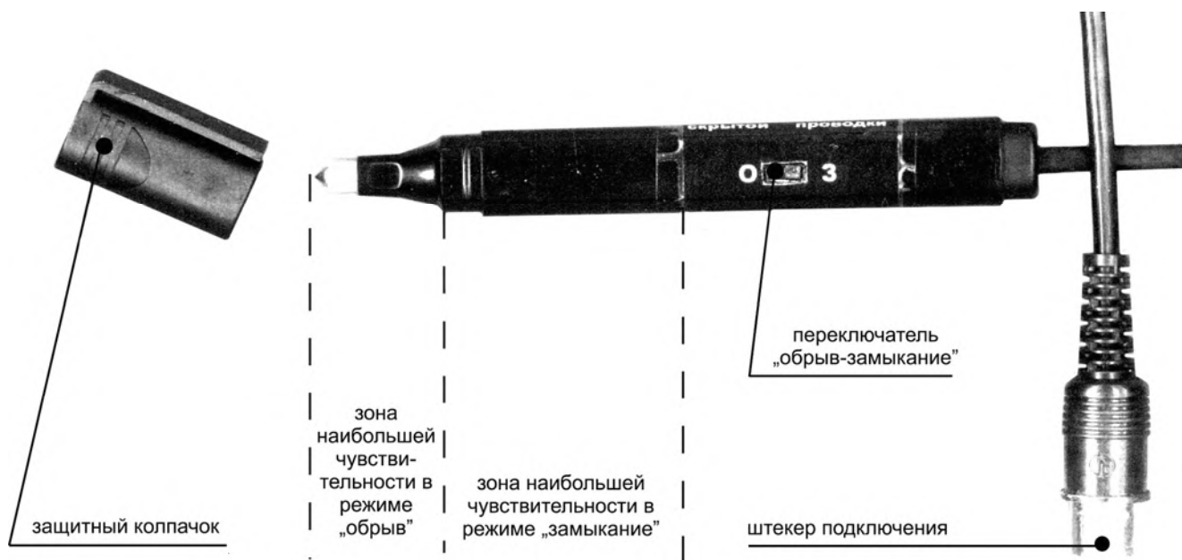
Рисунок 5.3.4.1 – Мини-датчик МД-01
