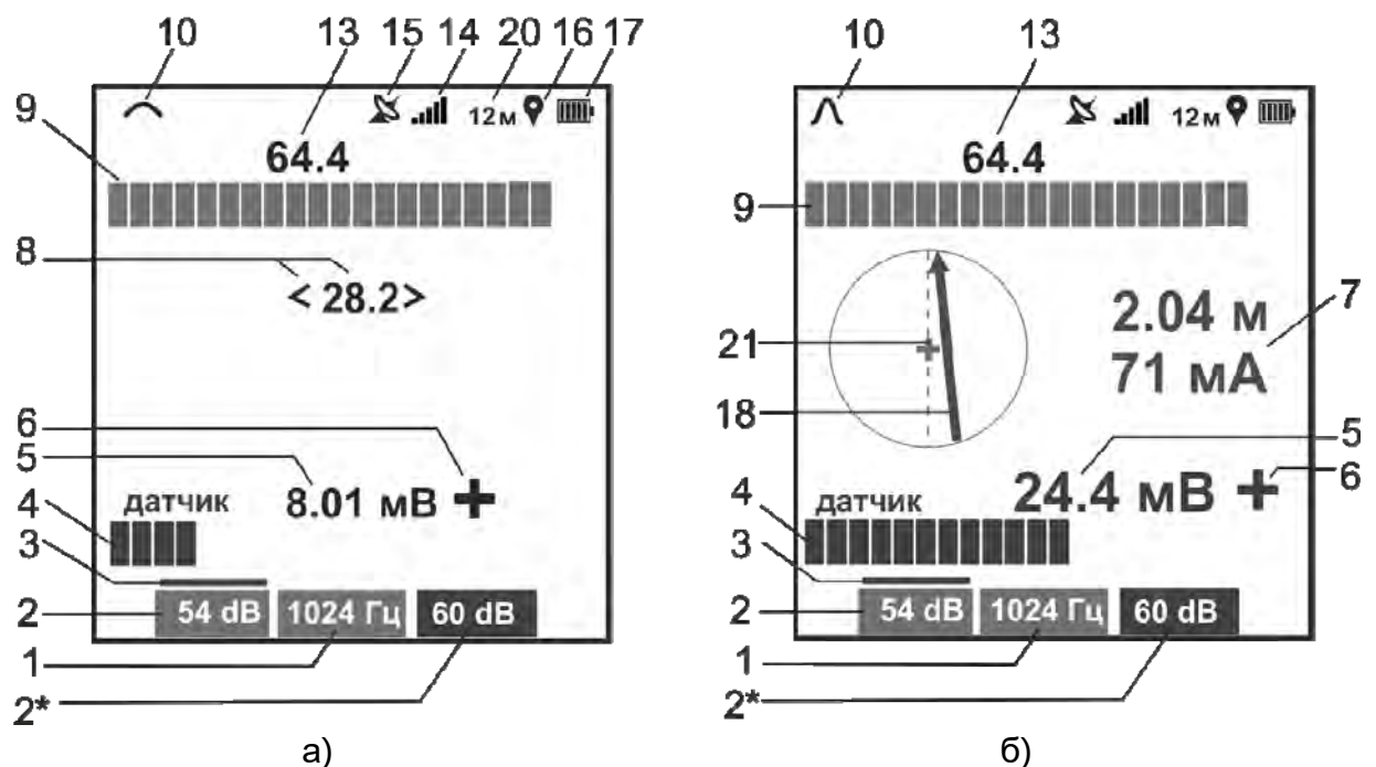
Рисунок 3.3 – Индикация приемника в режиме «ТРАССА-ДАТЧИК»
