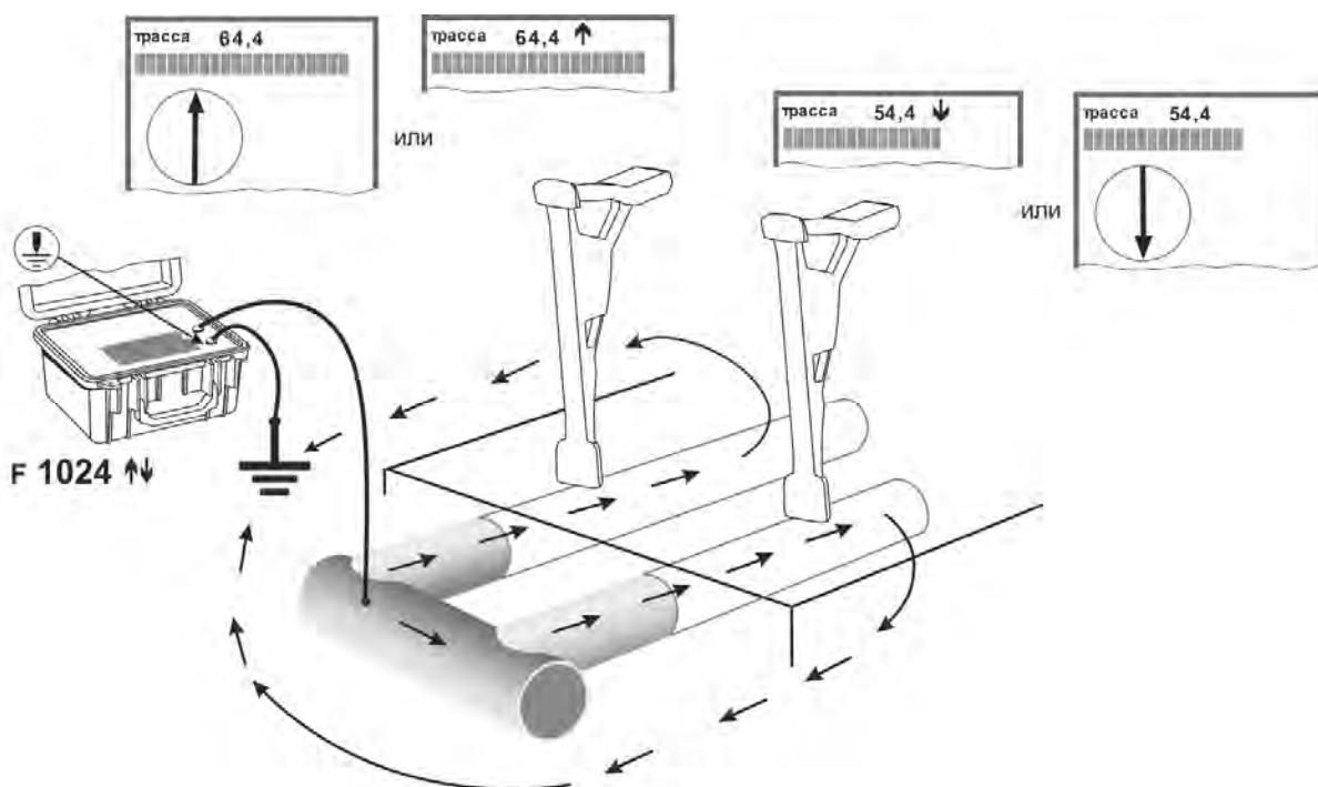
Рисунок 4.2.4б – Направление тока и показания приемника при гальванически связанных коммуникациях
