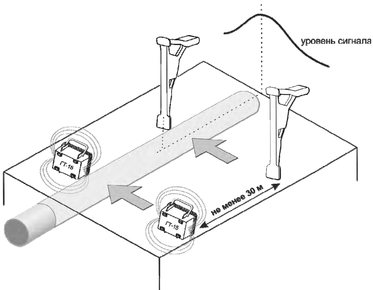
Рисунок 4.4.2 б – Обследование участков местности с помощью ГТ-15
