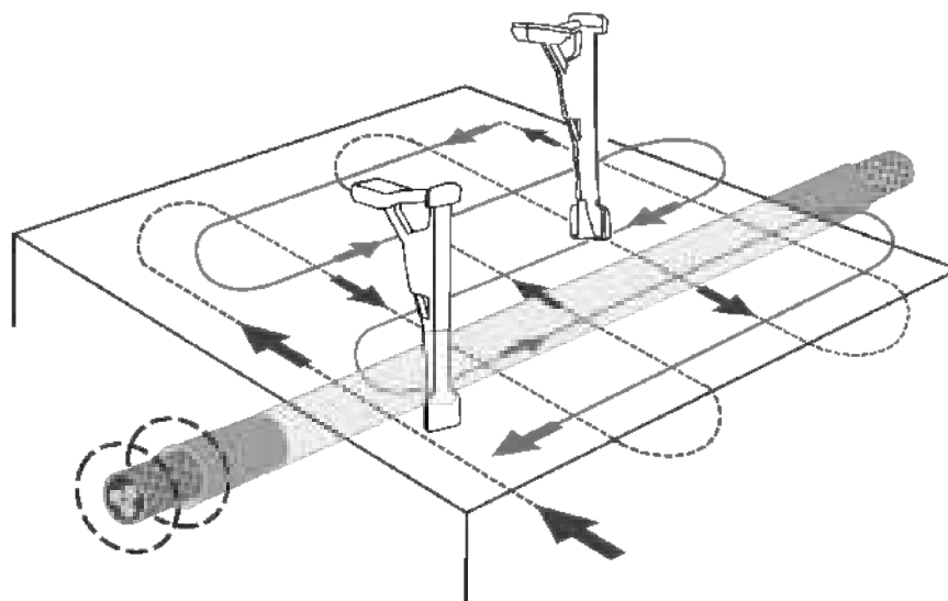
Рисунок 4.4.1 – Обследование участков местности без генератора
