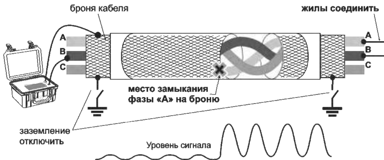
Рисунок 5.3.2 – Схема подключения и уровень сигнала при поиске замыкания жилы на броню
