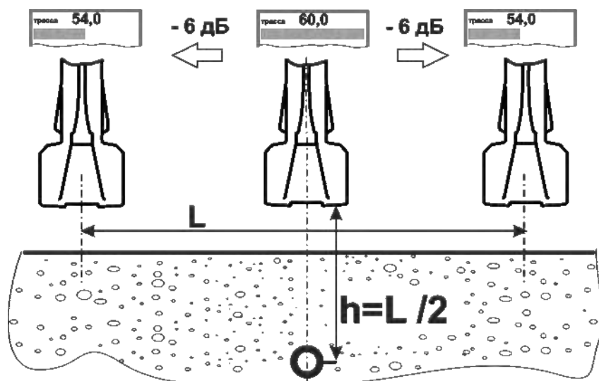
Рисунок 4.3.1 – Определение глубины залегания методом «-6дБ»
