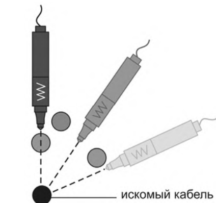
Рисунок 5.4.2 – Отбор жилы по минимуму сигнала
