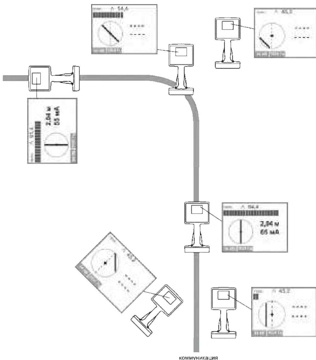
Рисунок 4.2.3а – Поиск с включенной функцией «КОМПАС»
