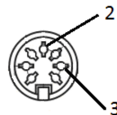
Рисунок 13.5.4 – Нумерация контактов гнезда «ДАТЧИК»
