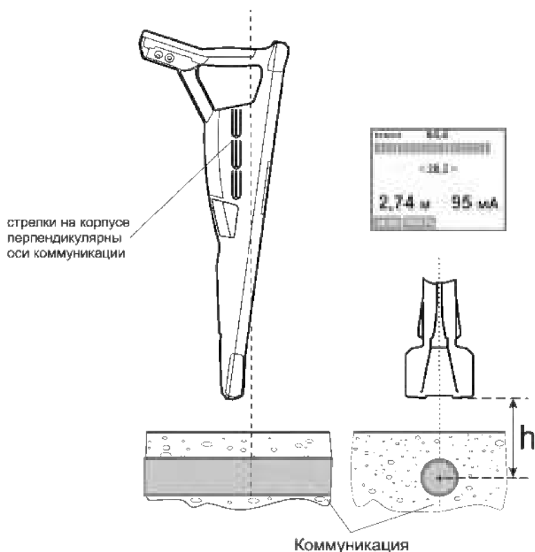
Рисунок 4.3 – Показания глубины залегания и тока
