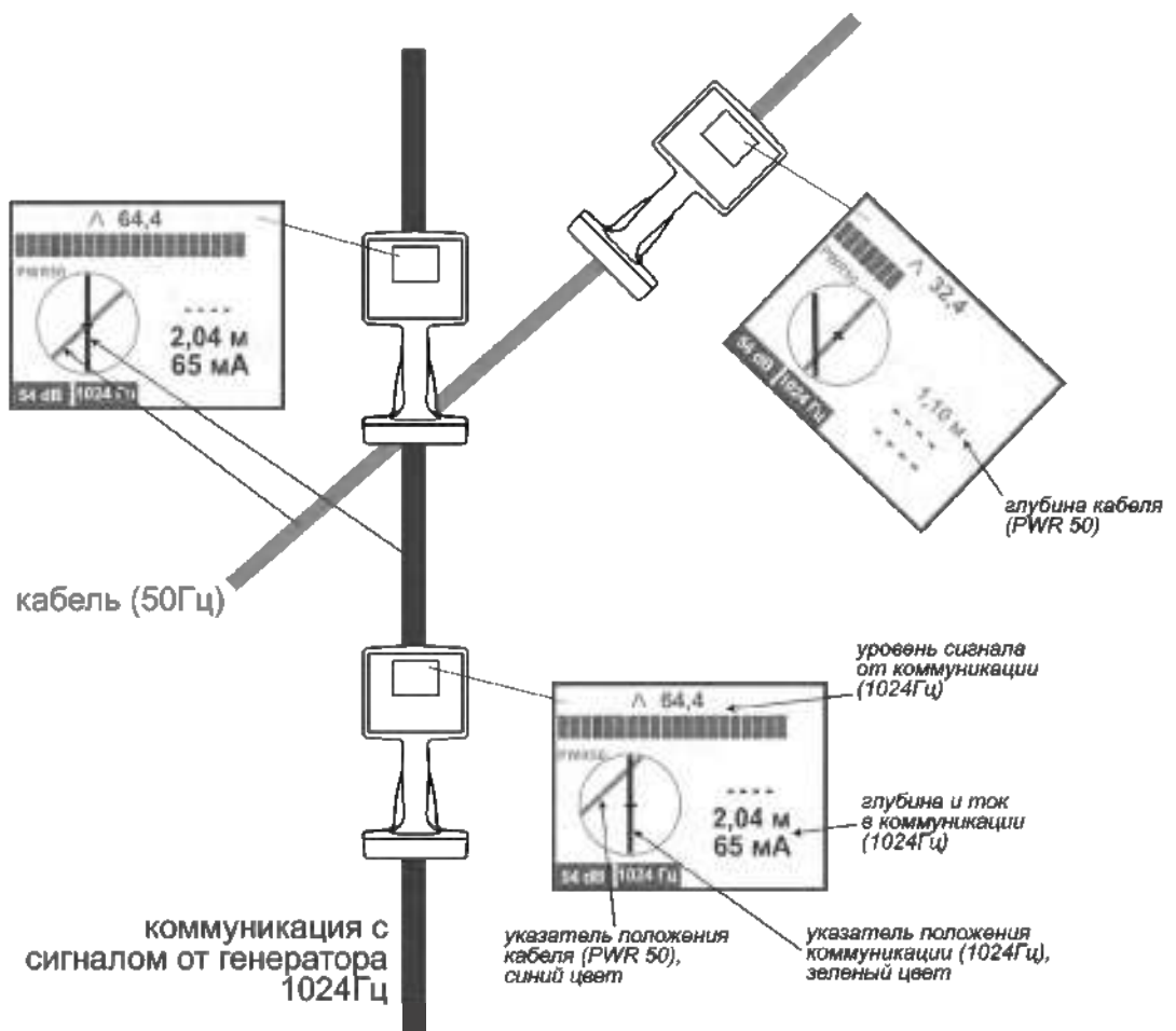
Рисунок 4.2.36 – Поиск с включенной функцией «Вторая линия»
