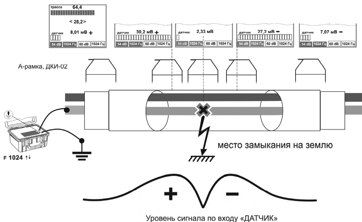
Рисунок 5.3.3.1 – Схема подключения и уровень сигнала при поиске повреждения изоляции с использованием датчиков контроля изоляции
