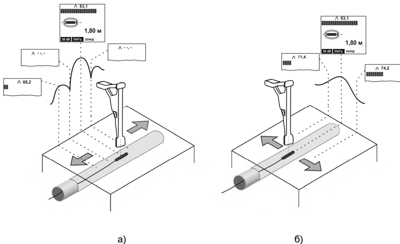
Рисунок 4.5.2 – Определение точного положения и глубины залегания зонда
